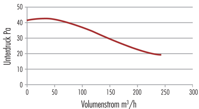
Leistungsdiagramm AirSpeedy®
